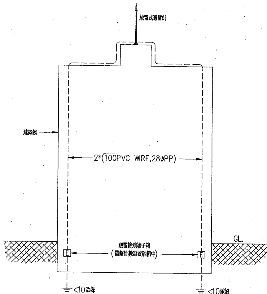
放電式避雷針裝置架構圖（一）
