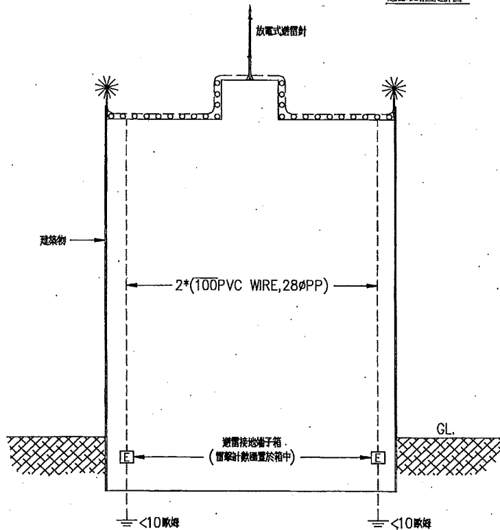
放電式避雷針裝置架構圖 (二)
