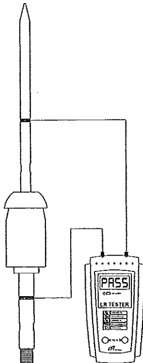
測試接線圖
